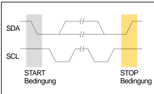
Bild 4: START- und STOP-Bedingung des I 2 C-Busses
