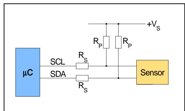
Bild 12: I 2 C-Bus-Anwenderschaltung für Sensortronics' digitale Drucksensoren
